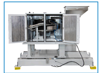
Integración de alimentadores vibratorios (de tazón) para componentes
