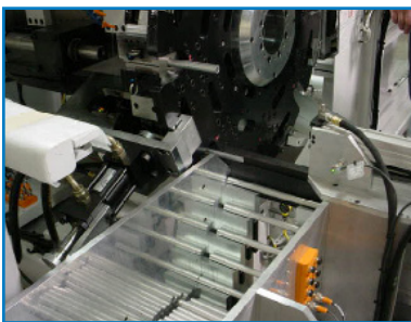
Tolvas ajustables para tubos
